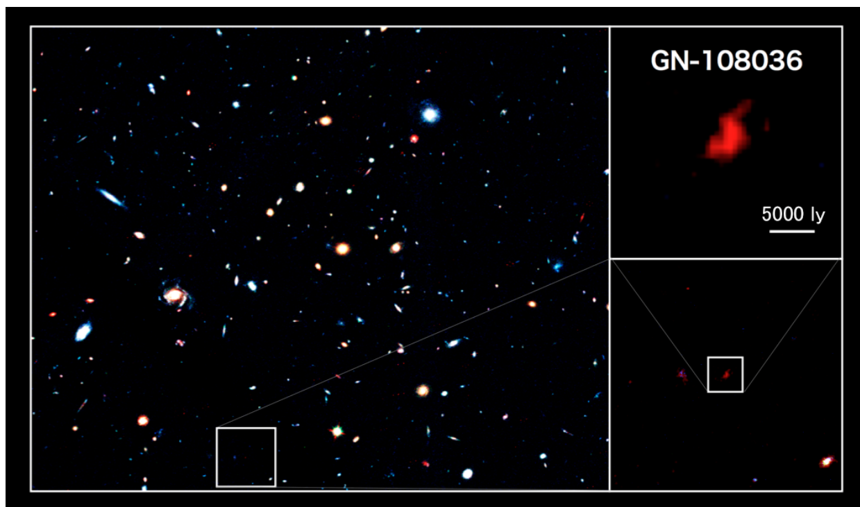
Figur 4. Det fjerneste objekt, man kender med sikkerhed, er en galakse GN-108036, der udsendte lys, da Universet var 750 millioner år gammelt. Den ses her i det lille kvadrat på en optagelse fra Hubble Ultra Deep Field og i de forstørrede billeder til højre.
